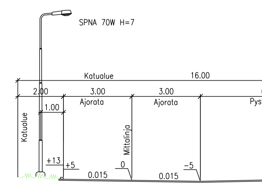
TAAVETINKATU TYYPPIPOIKKILEIKKAUS, AJORATA PLV 0 - 31
