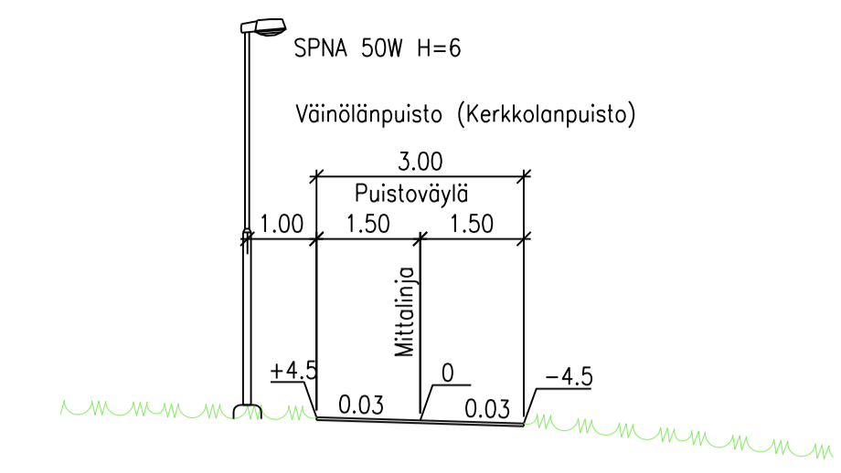
PUUSTOVÄYLÄ 1 (Väinölänpolku-Riihimäenkatu) TYYPPIPOIKKILEIKKAUS
