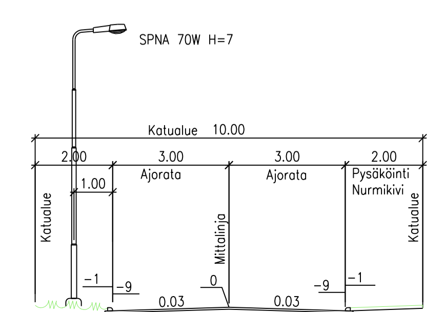
TAAVETINKATU TYYPPIPOIKKILEIKKAUS, AJORATA PLV 44 - 98
