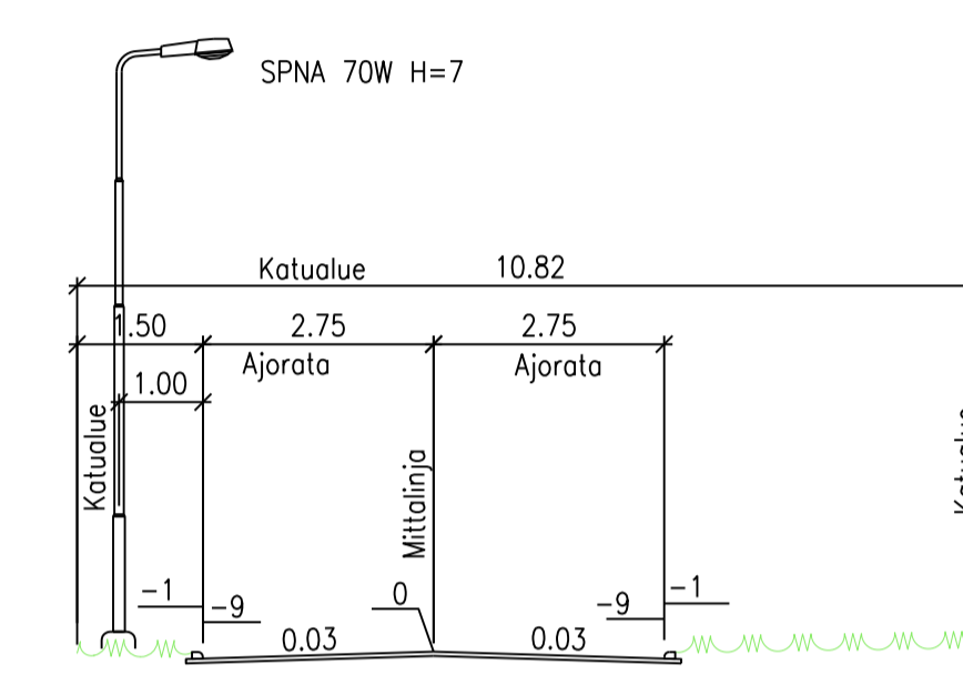
VÄINÖLÄNKATU TYYPPIPOIKKILEIKKAUS, AJORATA PLV 102 - 124
